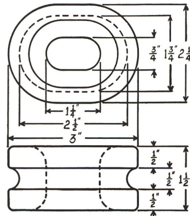
No. M6844 U. S. No. D6
