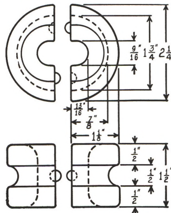
No. M6539 U. S. No. D2
